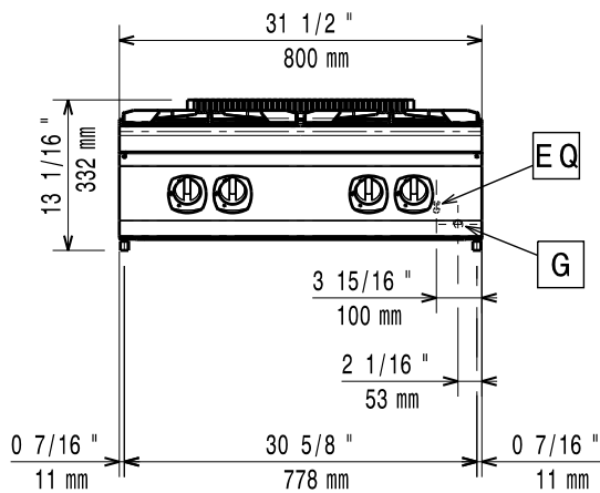
Alzado
